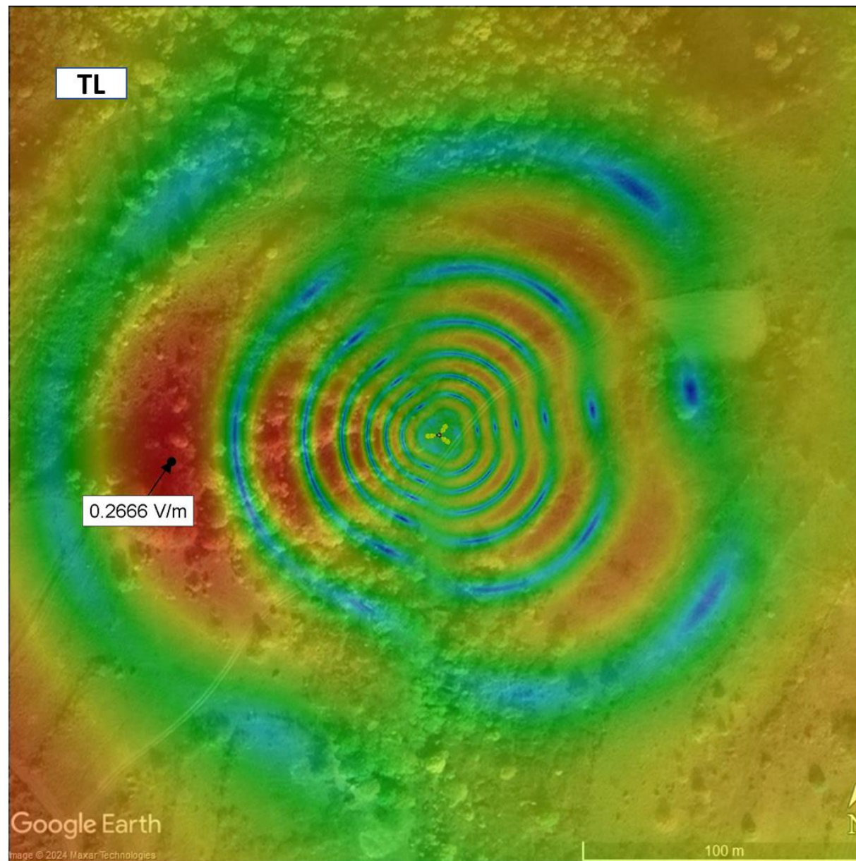
Слика 4.6. Јачина електричног поља на тлу када радио-систем LTE2100 оператора A1 Србија ради максималним капацитетом
