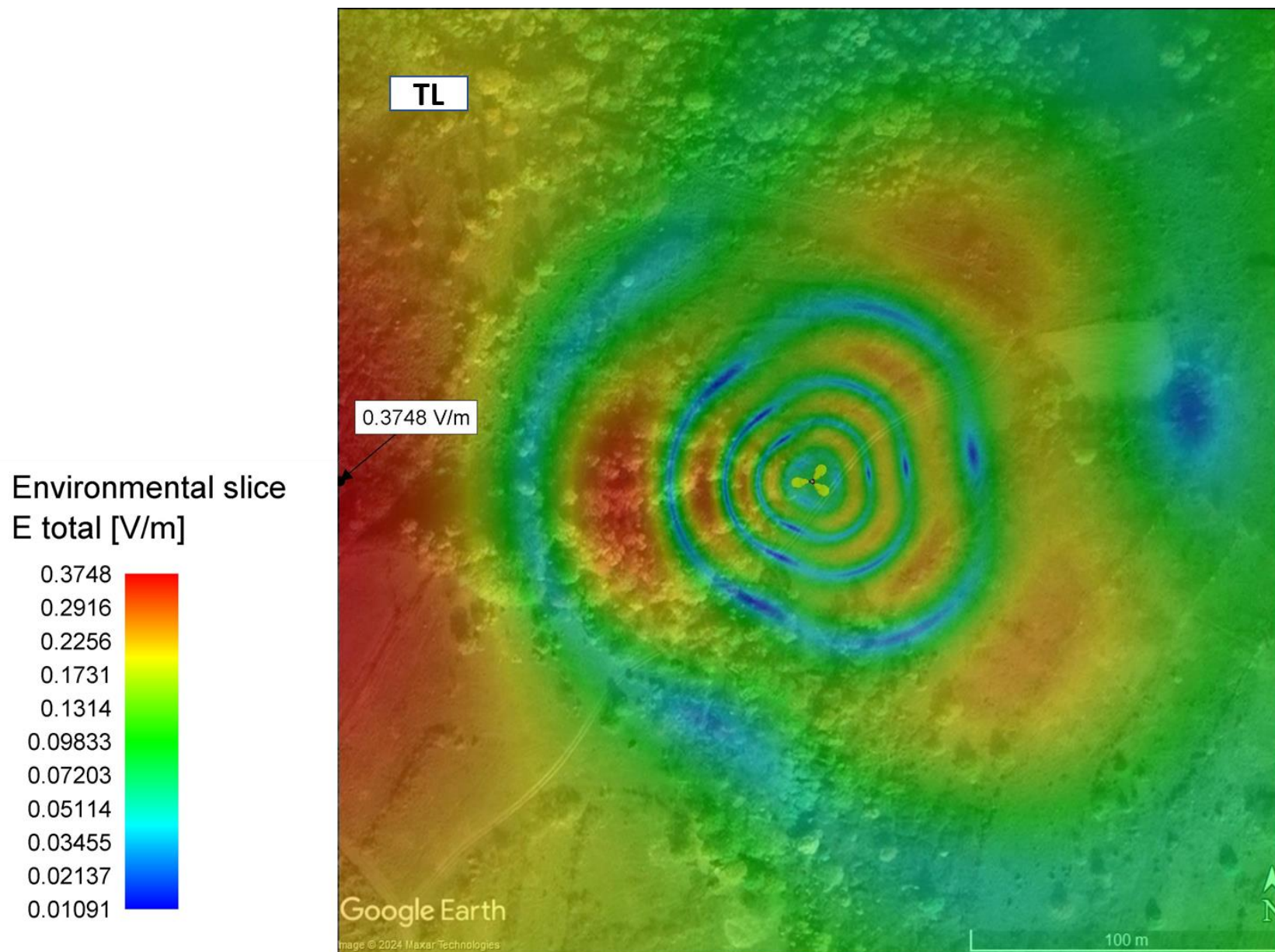
Слика 4.4. Јачина електричног поља на тлу када радио-систем LTE800 оператора A1 Србија ради максималним капацитетом
