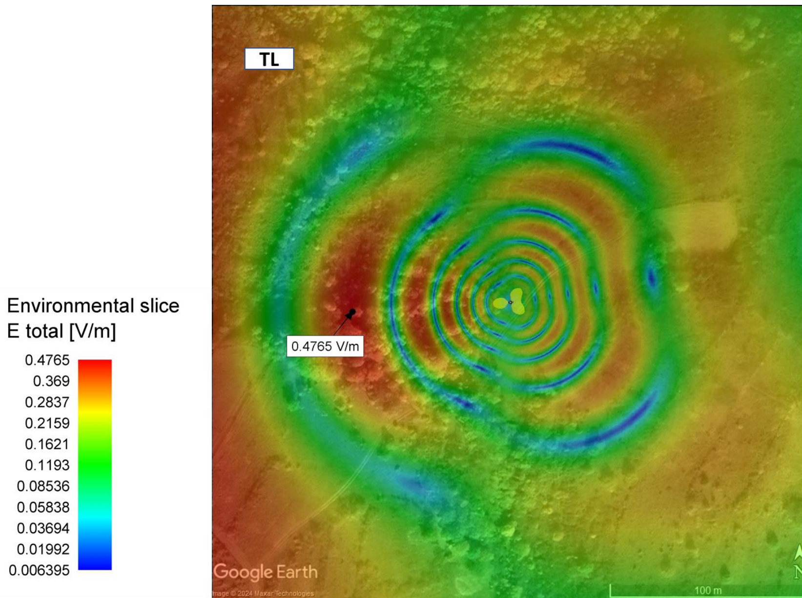
Слика 4.5. Јачина електричног поља на тлу када радио-систем LTE1800 оператора А1 Србија ради максималним капацитетом
