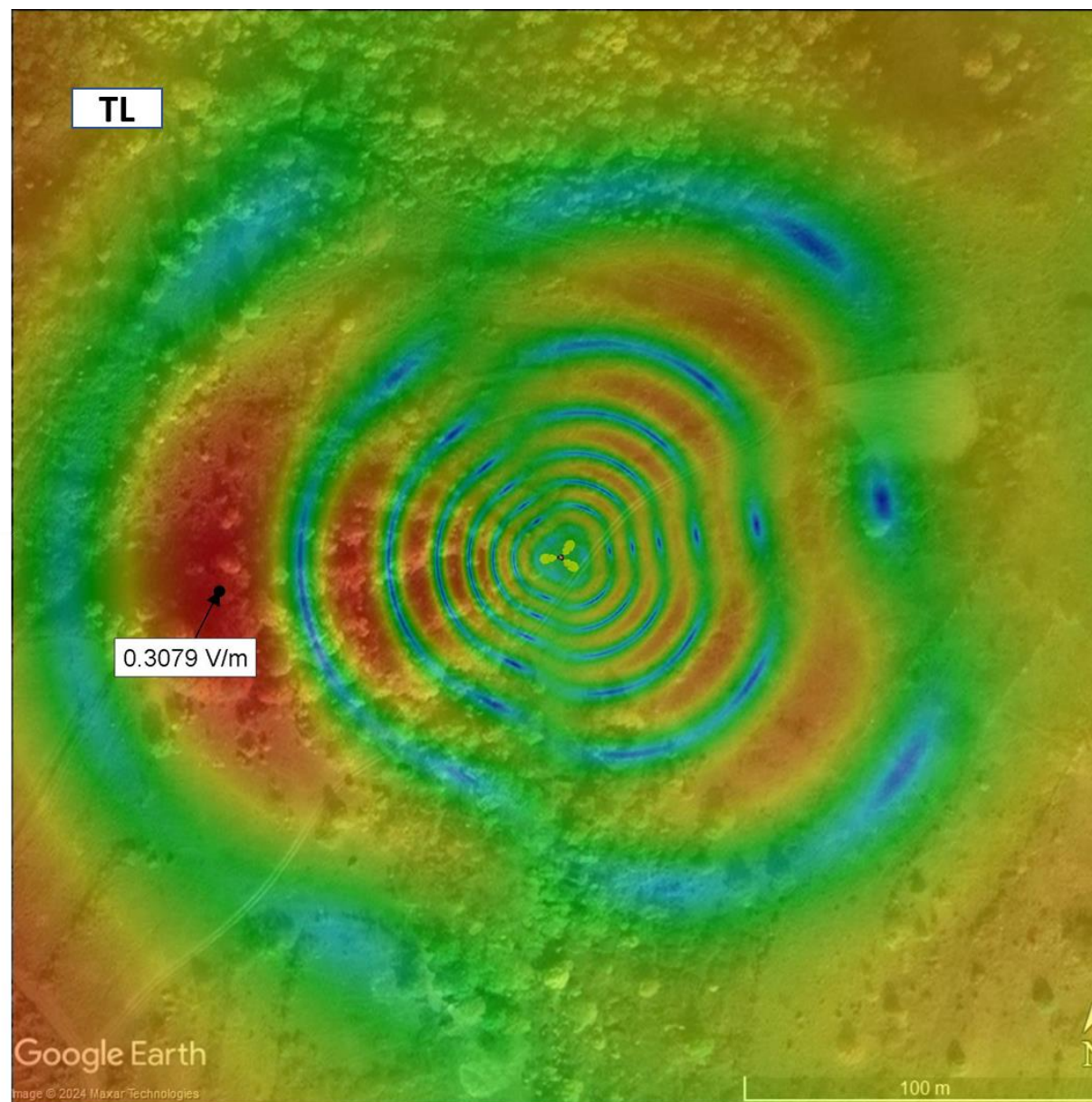
Слика 4.3. Јачина електричног поља на тлу када радио-систем UMTS2100 оператора А1 Србија ради максималним капацитетом
