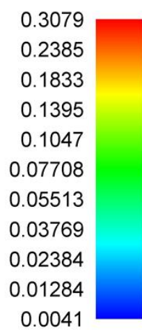
Слика 4.3. Јачина електричног поља на тлу када радио-систем UMTS2100 оператора А1 Србија ради максималним капацитетом
